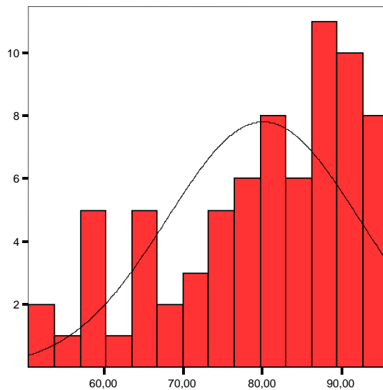
Comisia 1 - Chimie
