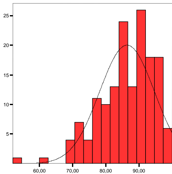
Comisia 1 - Fizica
