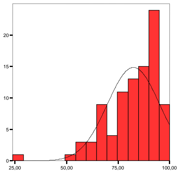
Comisia 1 - Matematica-Informatica
